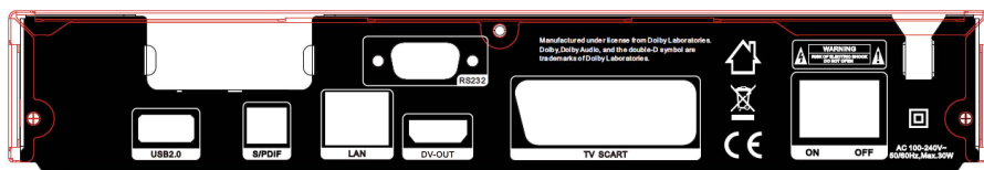
Zadný panel AB CryptoBox 750HD
