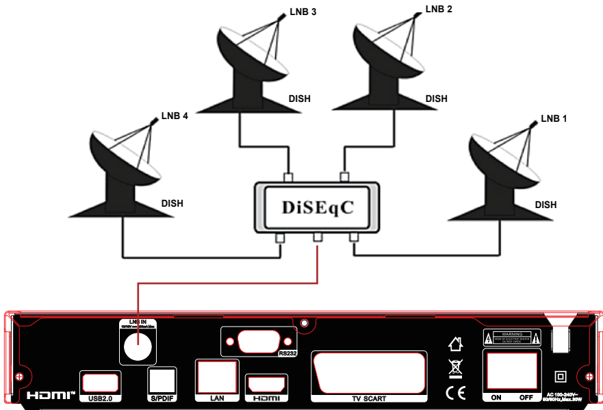
Obrázek 7. Připojení k LNB pomocí DiSEqC
