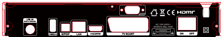
Zadný panel AB CryptoBox 700HD
