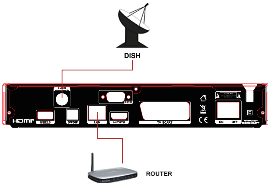
Obrázek 6. Připojení k LNB
