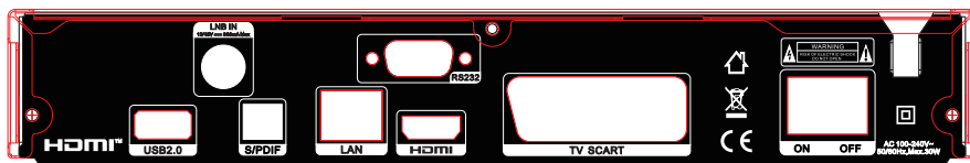
Zadnýpanel AB CryptoBox 740HD
