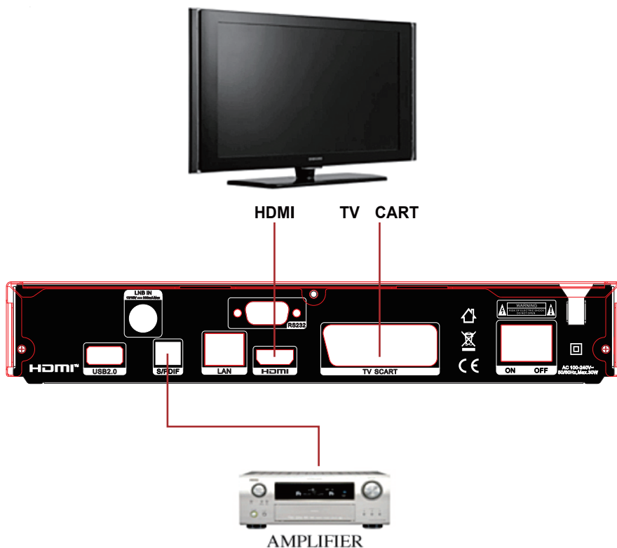
Obrázok 4. Pripojenie k TV a zosilňovaču
