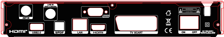
Abbildung 3. Rückplatte
